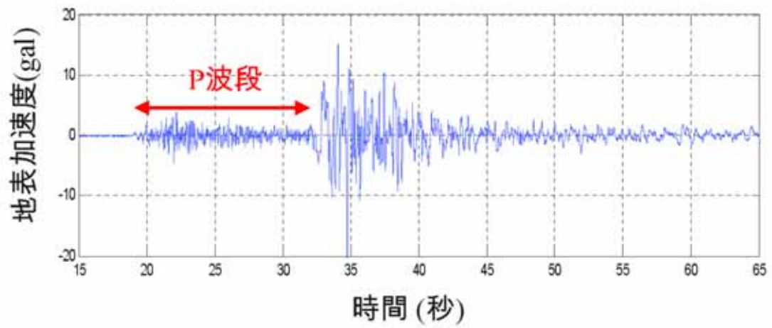
圖 1. 地震引發地表加速度之典型時間震波型態，圖中 P 波段即為 P 波與 S 波速度差造成之走時差（2010/11/21 花蓮地震 921 地震教育園區東西向測站紀錄）
