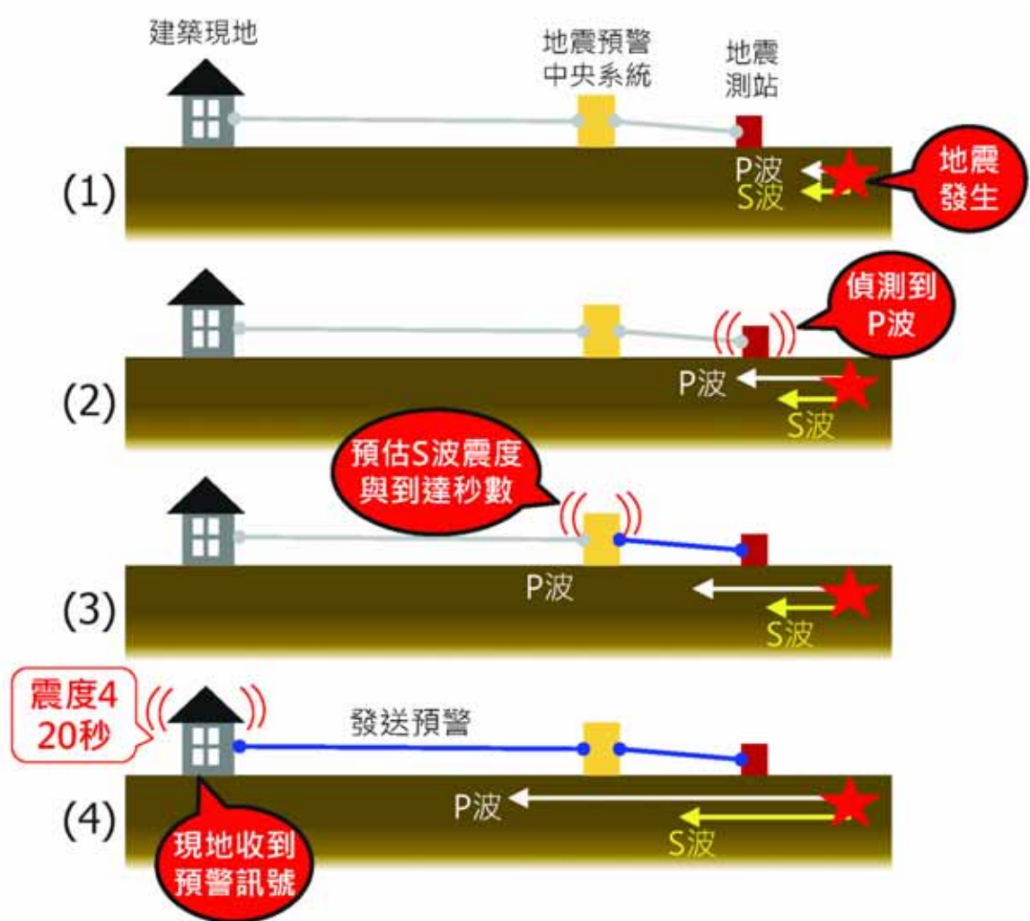
圖 2. 區域地震預警運作四階段示意圖
